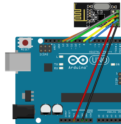
（圖九）連接方式概念圖
