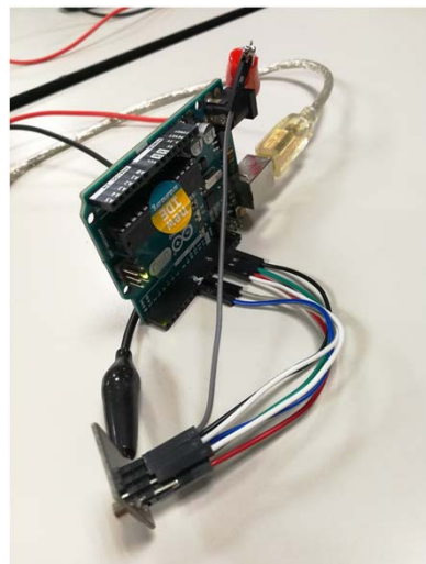
（圖七）板子和天線的連接方式
