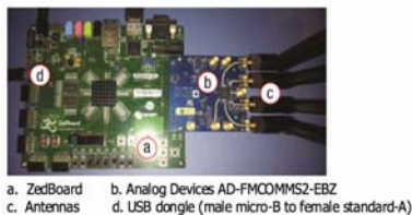
圖十一、ZedBoard架構介紹
